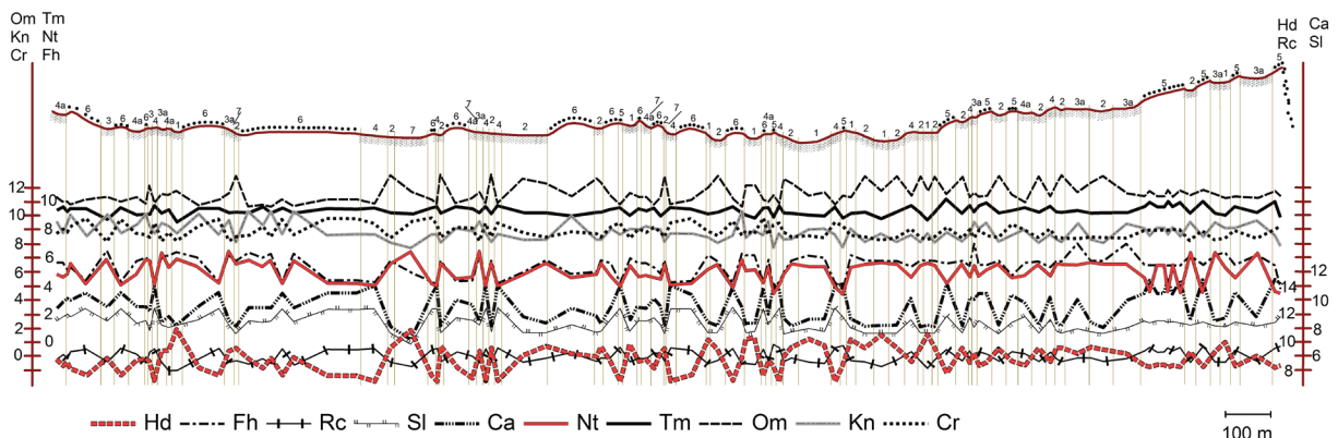
Рис. 2. Закономірності диференціації рослинних угруповань та показників екофакторів на екологічному профілі векторного типу Карабі-яйли. У дужках наведено мнемокоди біотопів (Didukh et al., 2016)
